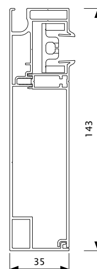
deep side channel (D)
